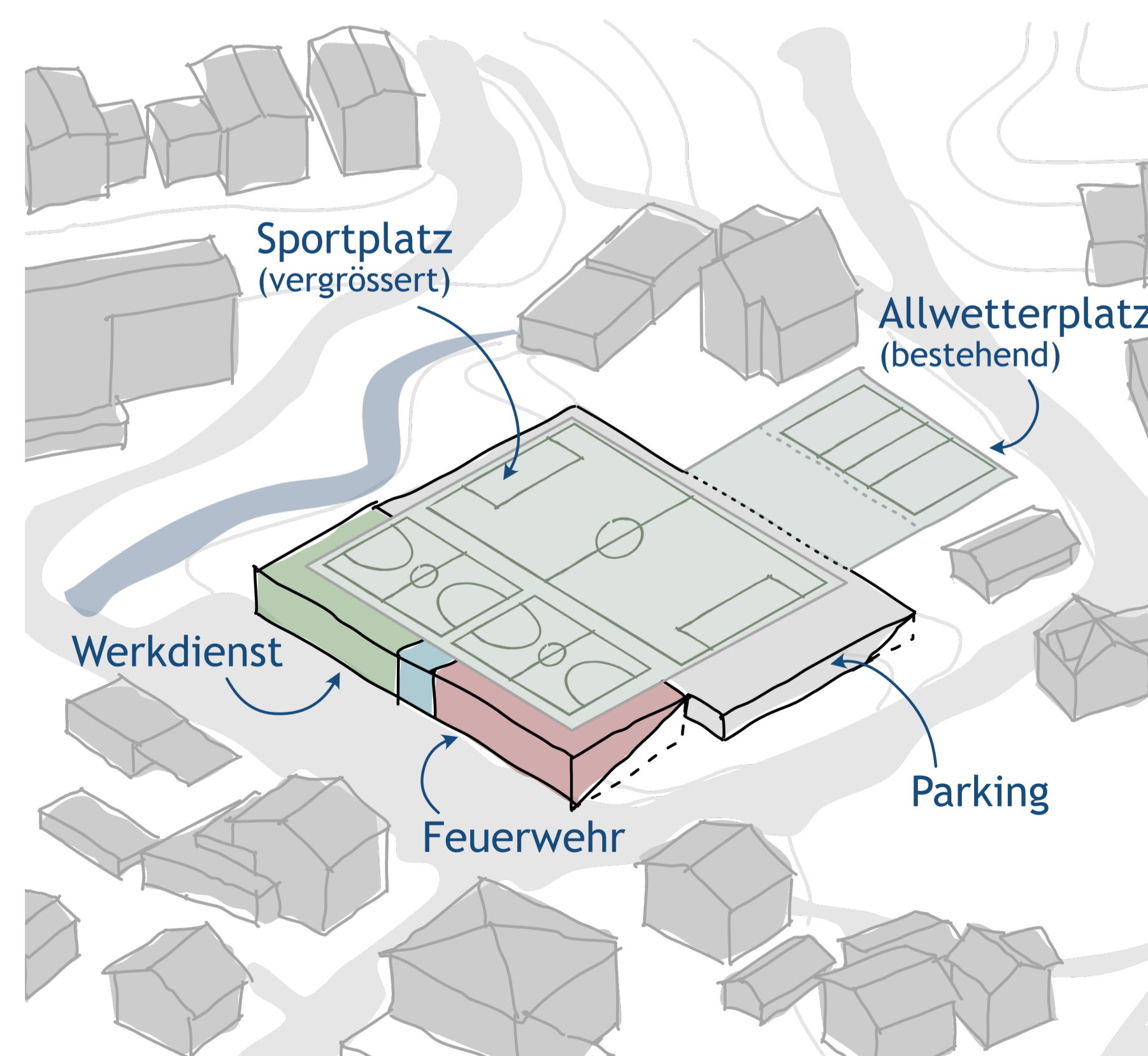
Variante 2: Feuerwehr, Werkdienst & Parking mit vergrössertem Sportplatz auf dem Dach
